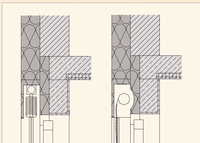
Tragender Universal-Ziegel-Raffstore-Rollladenkasten für Mauerstärke von 25 cm bis 30 cm
